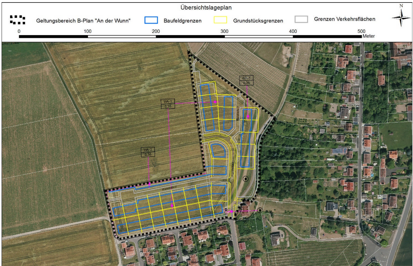
Abb. 2: Geltungsbereich der Baumaßnahme und Planung
